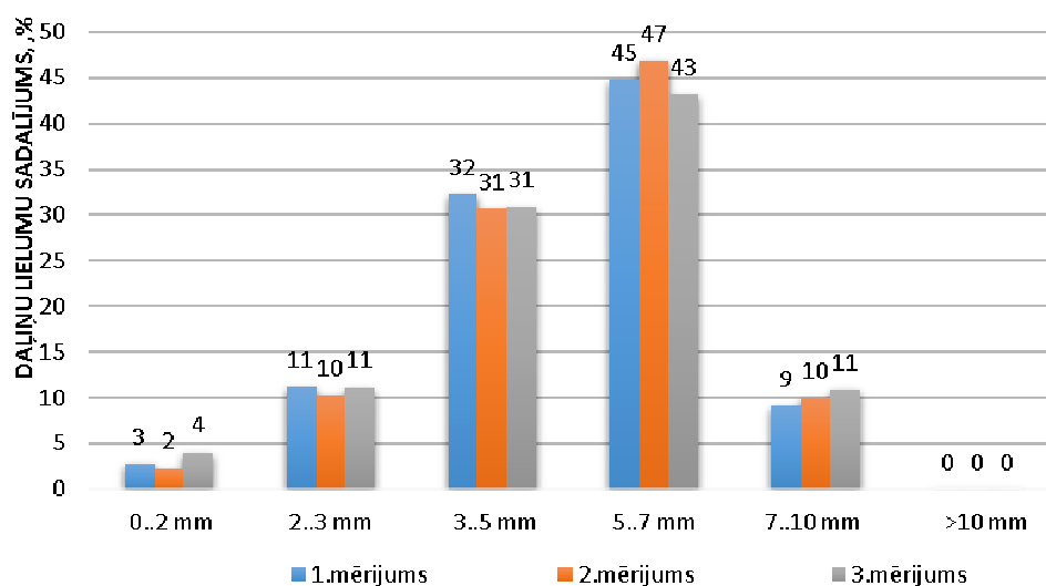
3. att. Smalcinātās masas daļiņu lielumu izkliede
