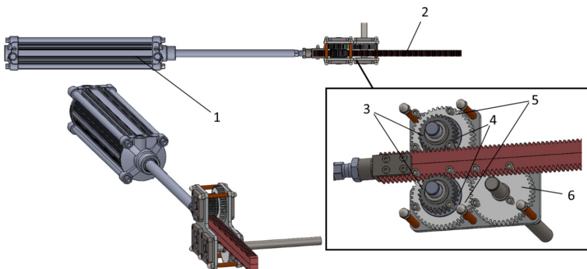
1. att. Pneimatiskais motors: 1 – pneimatiskais cilindrs; 2 – zobstienis; 3 – brīvrumba; 4 – starplika; 5 – zobrats; 6 – pārnesekārbas zobrats
