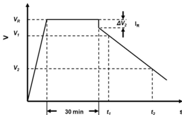
1. att. IEC standarta superkondensatora testēšanas metode
