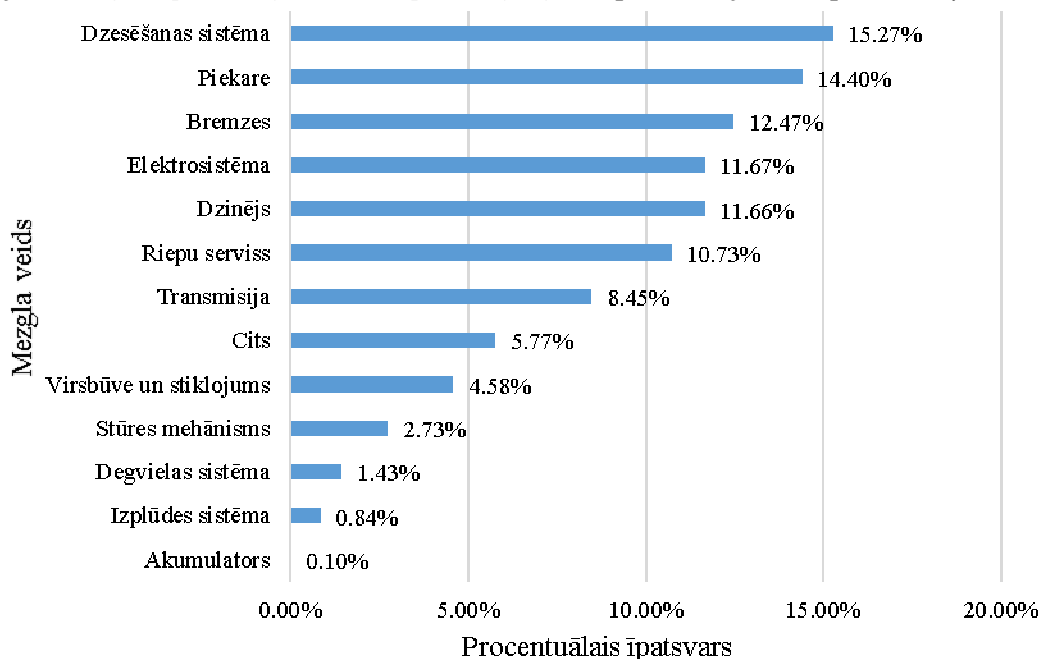
5. att. Remontu un apkopju īpatsvars 2019. gadā pēc mezglu veida specififikācijai Vieglais plašlietojuma – kompaktais furgons
