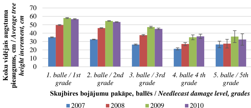
3.10. att. Skujbires ietekme uz koku vidējo augstumu pieaugumu ( \pm standartklūda) Ogres stādījumā/ Fig. 3.10. Effect of needlecast on height increment ( \pm SE) in the Ogre trial
