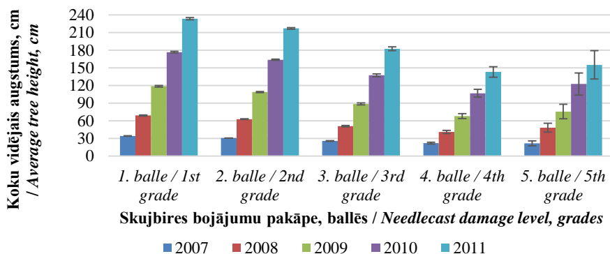
3.11. att. Skujbires ietekme uz koku vidējo augstumu ( \pm standartklūda) Ogres stādījumā/ Fig. 3.11. Effect of needlecast on average tree height ( \pm SE) in the Ogre trial
